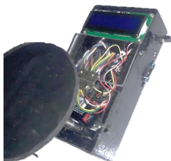
FIGURA 6. Protótipo final com disco de apoio acoplado (Autoria própria).
